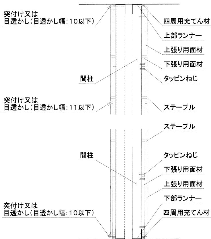
図22 上下端部詳細図(間柱を独立配置とする場合)
